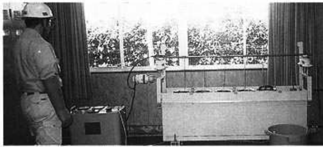
ヘルメットの耐圧試験
